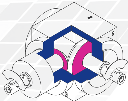
Abbildung 7.2.14-2; Getriebeseiten
