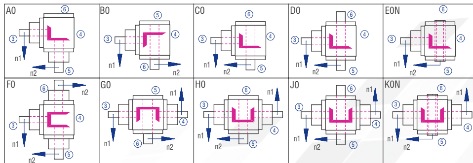
Abbildung 7.2.14-1; Bauarten
