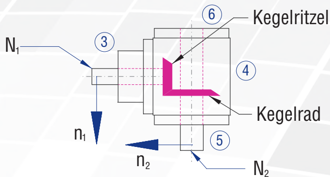
Abbildung 7.2.14-3; Wellenbezeichnungen
